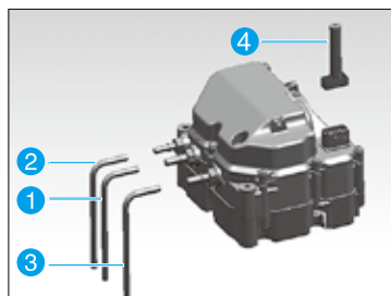
1. 回流到尿素管的管路 2. 流入后处理给料单元的管路网 3. 流入后处理喷射单元的管路 4. 电源线
